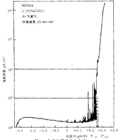
图1 参考的阳极极化曲线
