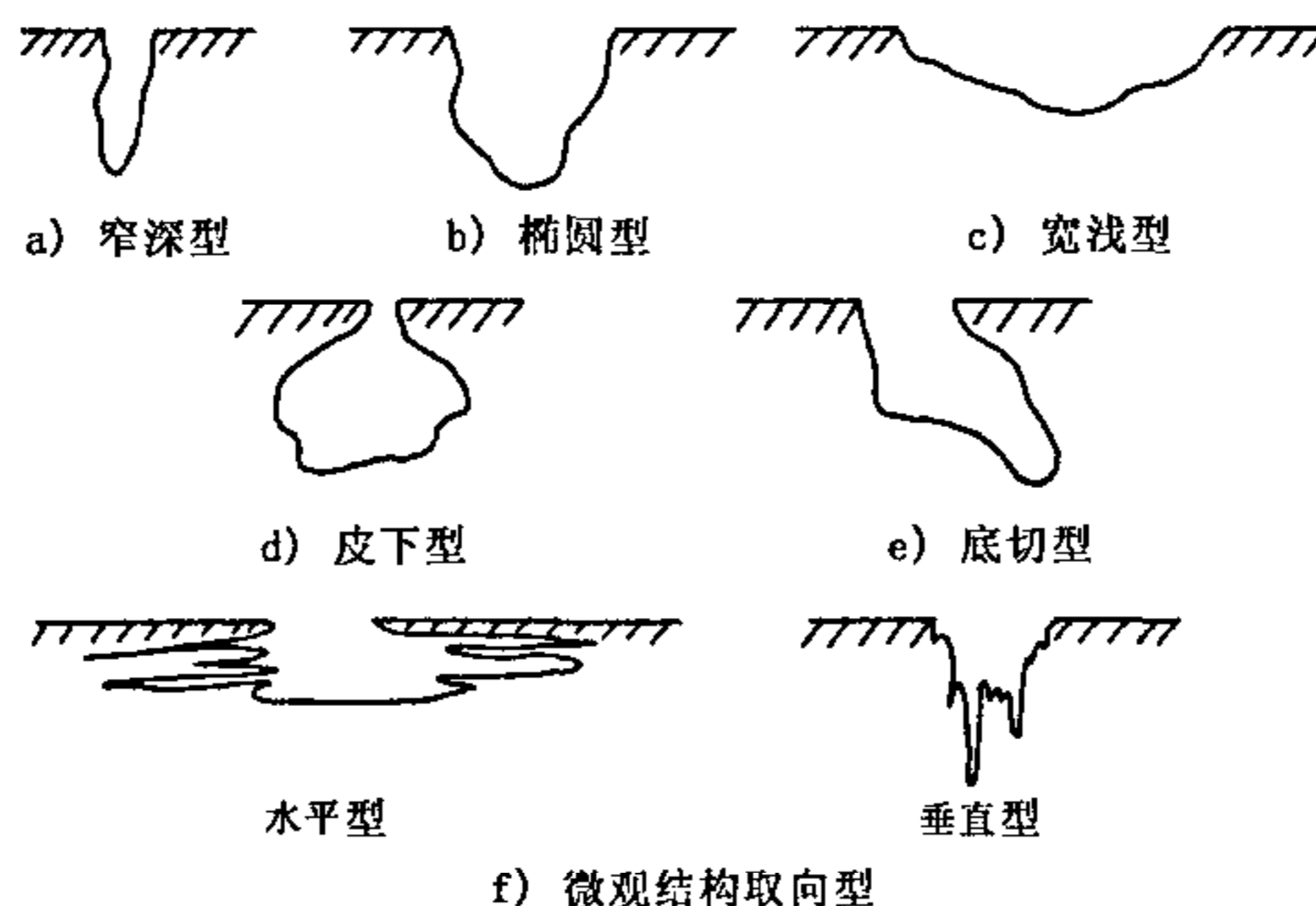
图1 蚀坑的不同横截面形状
