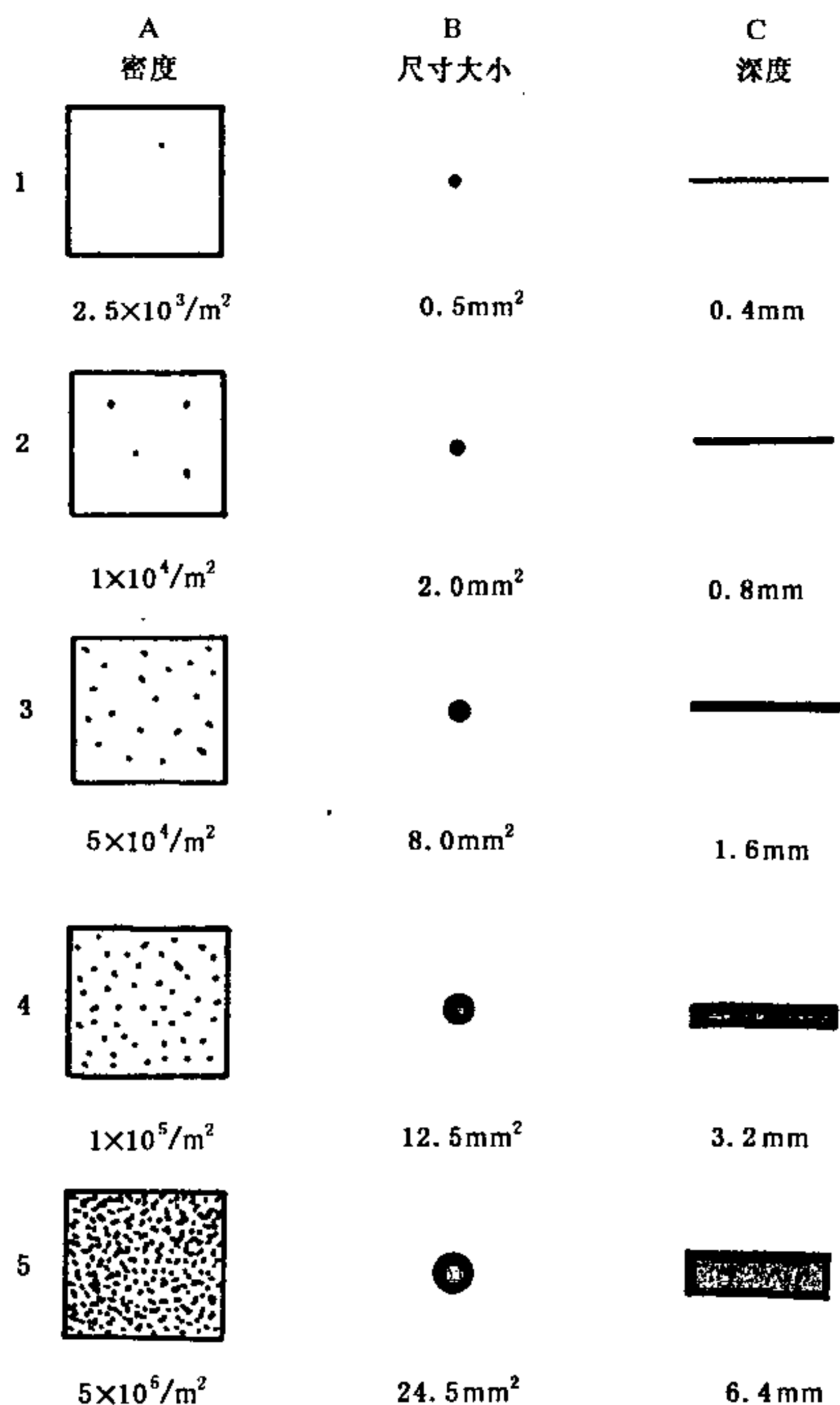
图 2 蚀坑的标准评级图
